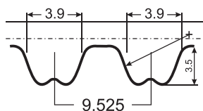
Профиль ремней ГРМ 2108-1006040 и 2112-1006040
