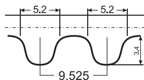
Профиль ремней ГРМ 21126-1006040
