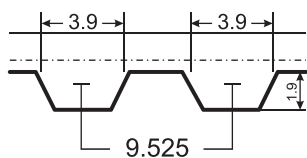
Профиль ремней ГРМ 2105-1006040
